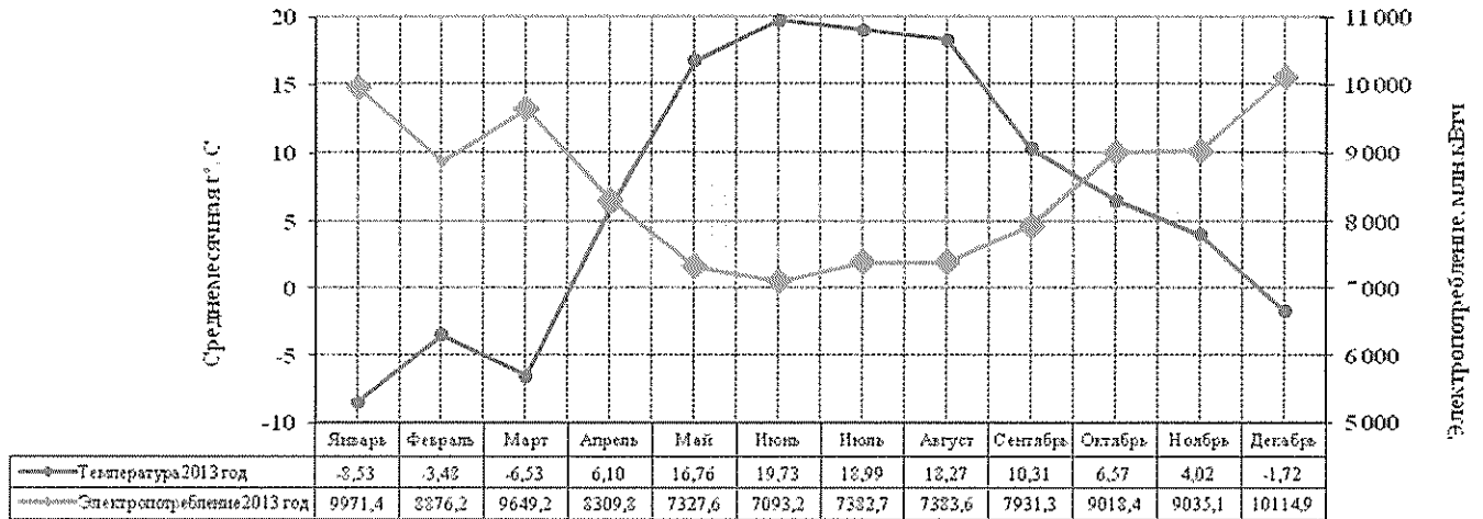
Температура наружного воздуха °С, Электронотребление Московского региона 2013 г.
