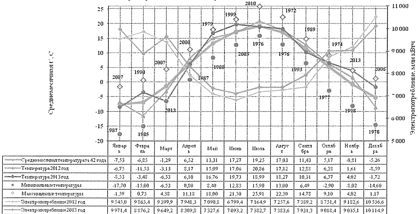
Изменение среднемесячной максимальной и минимальной °С за период 1972-2013 Электронотребление Московского региона 2012-2013 гг.
